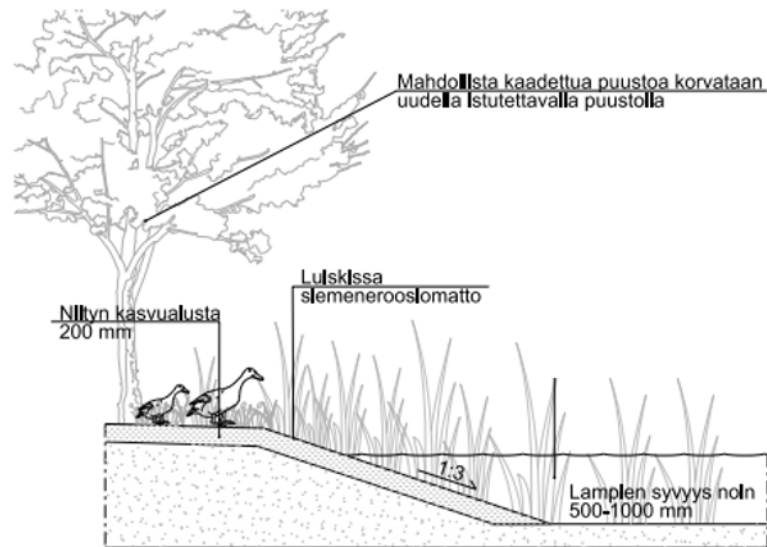
Periaateleikkaus lammen reunasta 1:50
