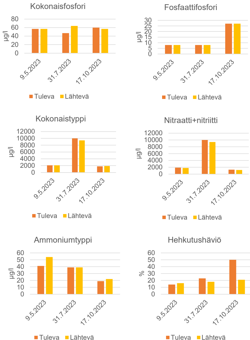
Kuva 11. Risupakanjoen alimmaiseen, vuonna 2022 rakennettuun kosteikkoon tulevan ja lähtevän veden näytetuloksia vuodelta 2023. Kosteikkoketjun seuranta jatkuvatoimisesti on aloitettu syksyllä 2024.
