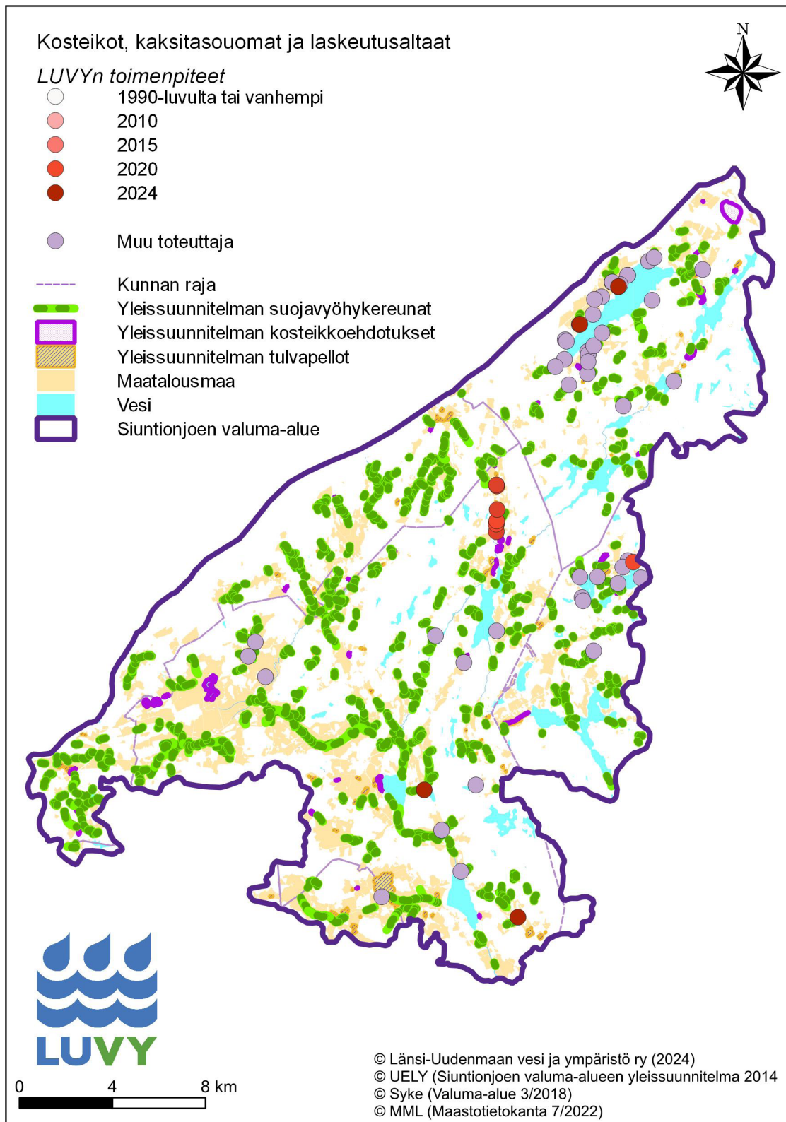
Kuva 10. Siuntionjoen valuma-alueelle rakennetut kosteikot, kaksitasouomat ja laskeutusaltaat. Kartassa on lisäksi valuma-alueen yleissuunnitelman (Nyqvist & Vuorinen 2014) suojavyöhyke- ja kosteikkoehdotukset sekä tulvapeltoalueet.
