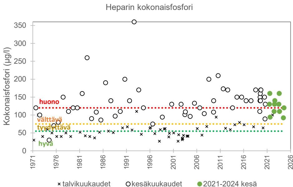
Kuva 16. Heparin kokonaisfosforipitoisuuden kehitys 1971–2023. Katkoviivat kuvaavat ekologisen tilaluokan rajoja. Tehokalastusvuodet ovat vihreillä symboleilla.
