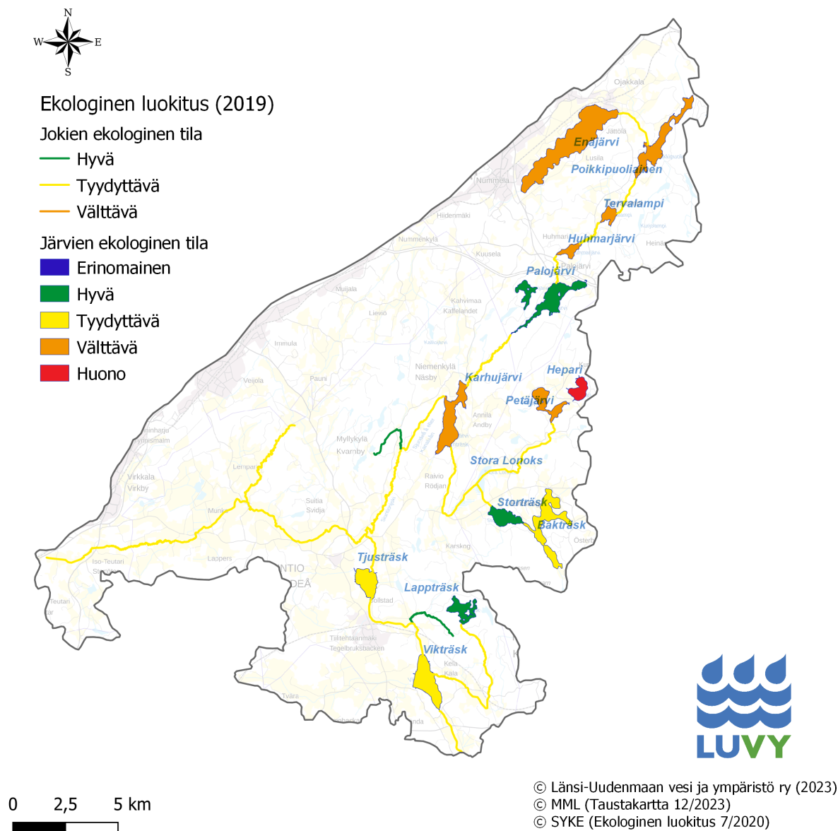
Kuva 3. Siuntionjoen ja sen järvien ekologinen tila.
