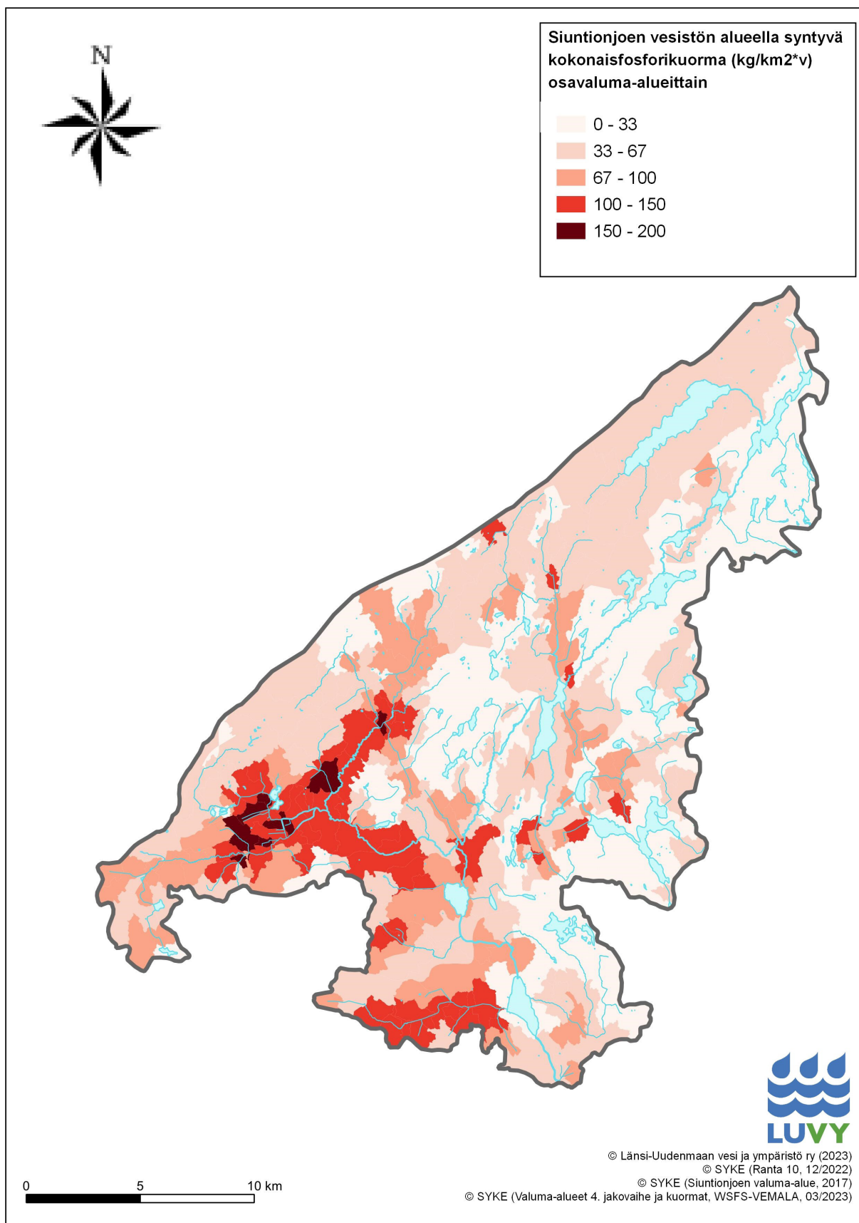
Kuva 6. Siuntionjoen kokonaisfosforikuormitus osavaluma-alueittain ympäristöhallinnon VEMALA-mallilla arvioituna.
