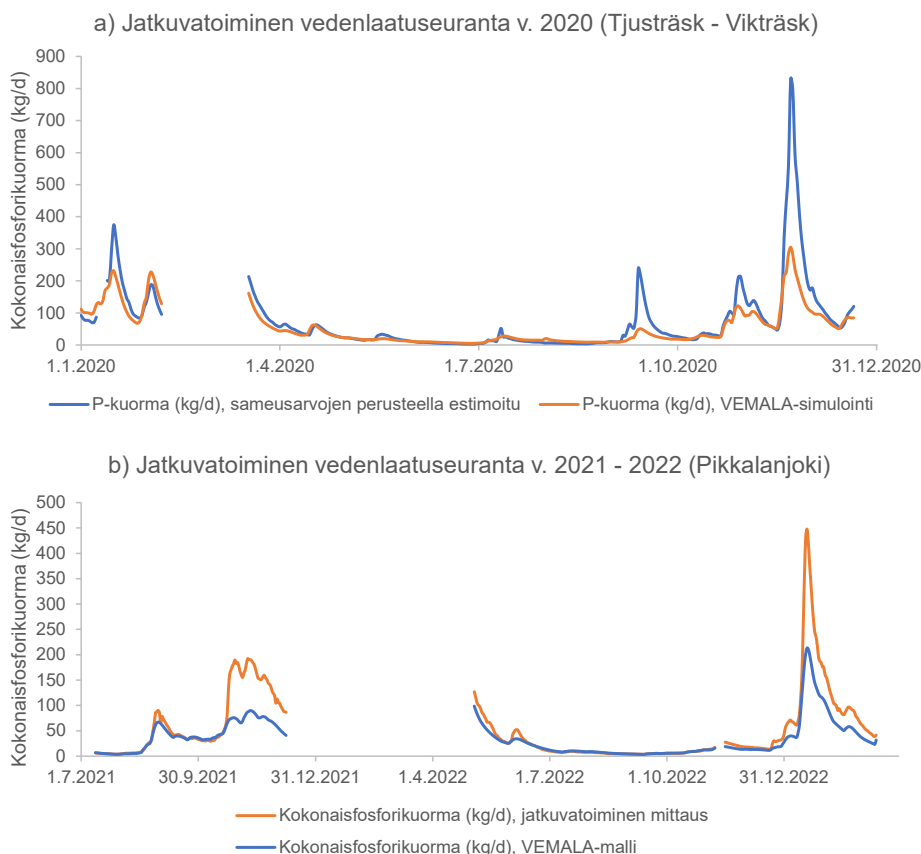
Kuva 26. Sameusarvojen perusteella estimoidut ja VEMALA-mallinnuksen simuloimat kokonaisfosforikuormat Tjusträskin ja Vikträskin välisellä mittausspaikalla vuonna 2020. Mittauksessa oli jäätälanteen vuoksi lyhyt tauko keväällä 2020.
