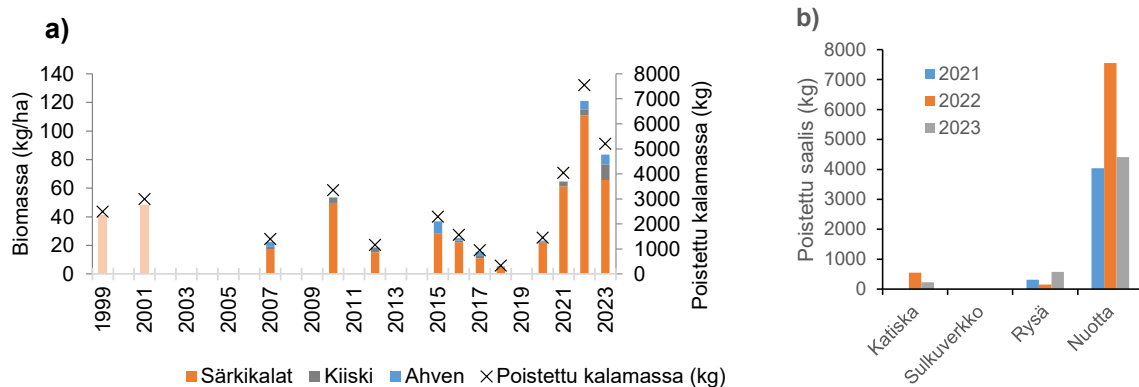
Kuva 14. a) Heparin hoitokalastussaaliit vuosina 1999–2023 ja b) vuosien 2021–2023 tehokalastusvaiheen saalis pyydyksittäin.
