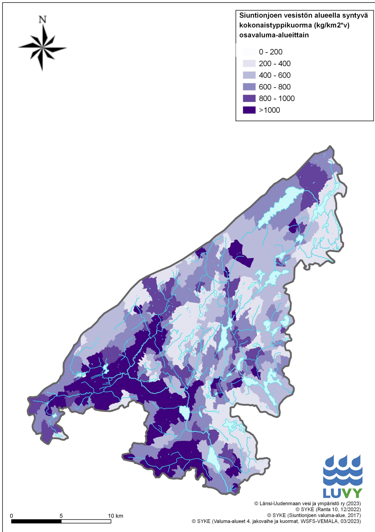
Kuva 7. Siuntionjoen kokonaistypikuormitus osavaluma-alueittain ympäristöhallinnon VEMALA-mallilla arvioituna.
