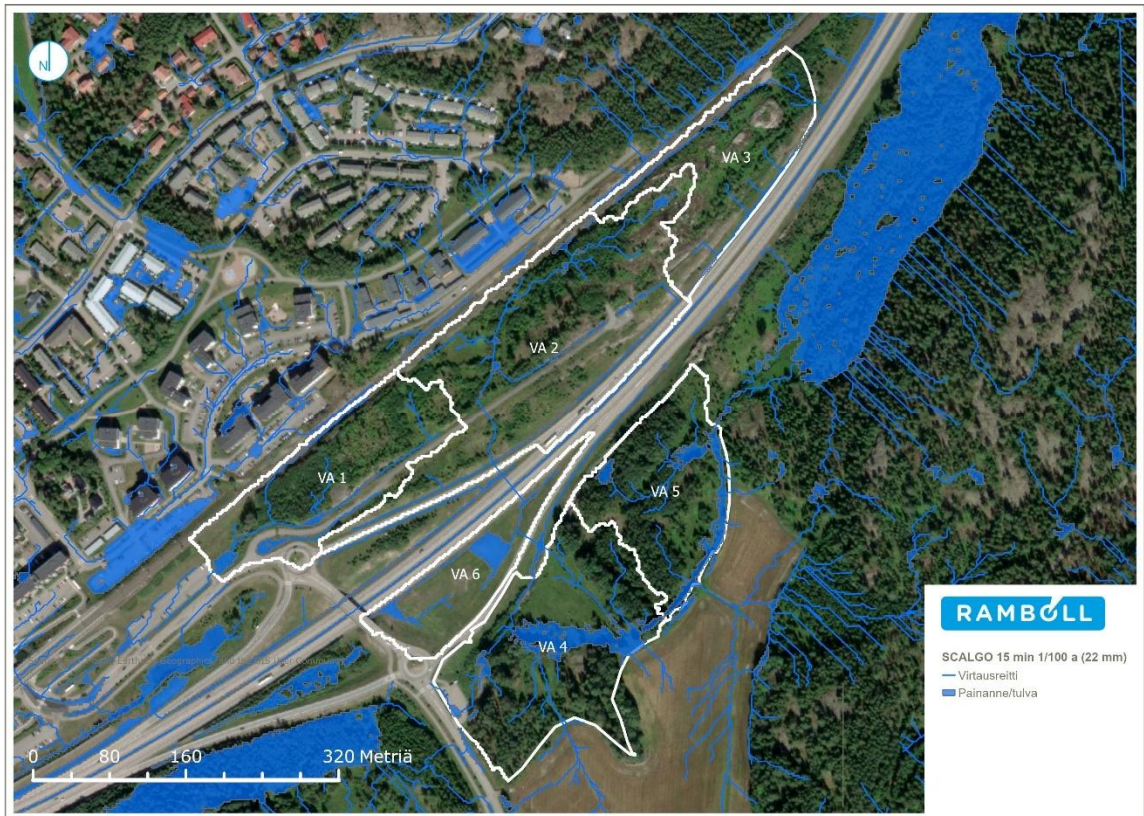
Kuva 9: Pintavaluntareitit ja osavaluma-alueiden rajat, nimet ja tulva-alueet nykytilanteessa (15 min sade 1/100 a) (Lähde: SCALGO).
