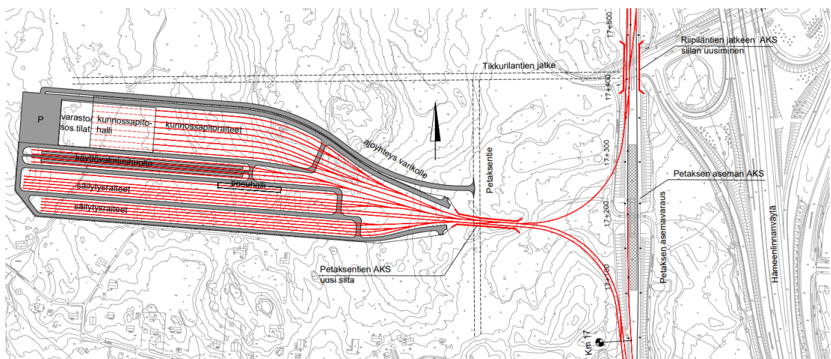
Kuva 18. Alustava suunnitelma Petaksen varikosta 80 junayksikölle (Väylävirasto 2020a).
