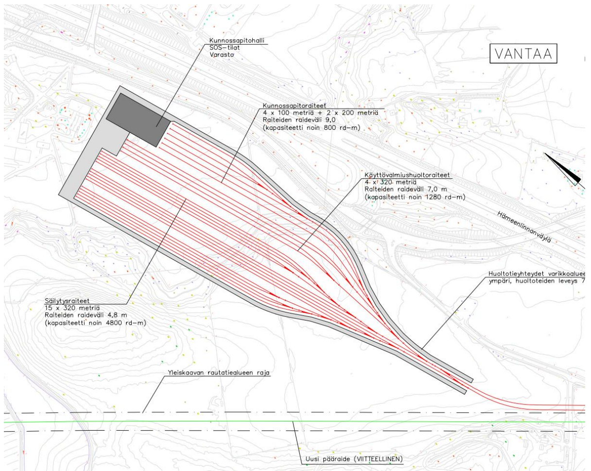
Kuva 19. Alustava suunnitelma Keimolan varikosta (mitoitus noin 80 junayksikköä).
