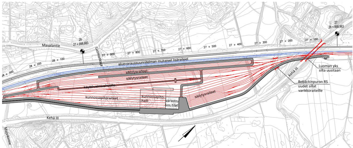
Kuva 16. Alustava suunnitelma Luoman varikosta noin 80 junayksikölle (Väylävirasto 2020a).
