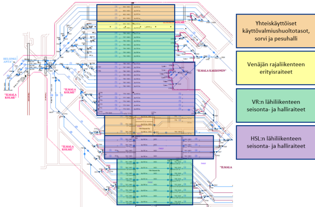
Kuva 5. Raiteiden pääsääntöiset käyttötarkoitukset Ilmala kolme -alueella (Väylävirasto 2020b).
