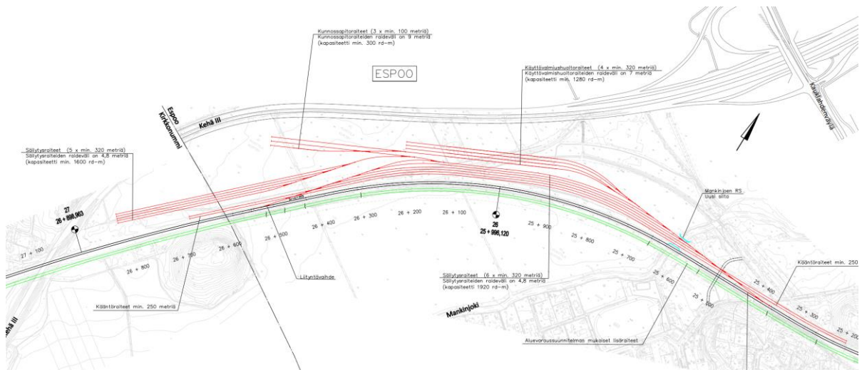
Kuva 15. Alustava suunnitelma Mankin varikosta (mitoitus noin 60 junayksikköä).
