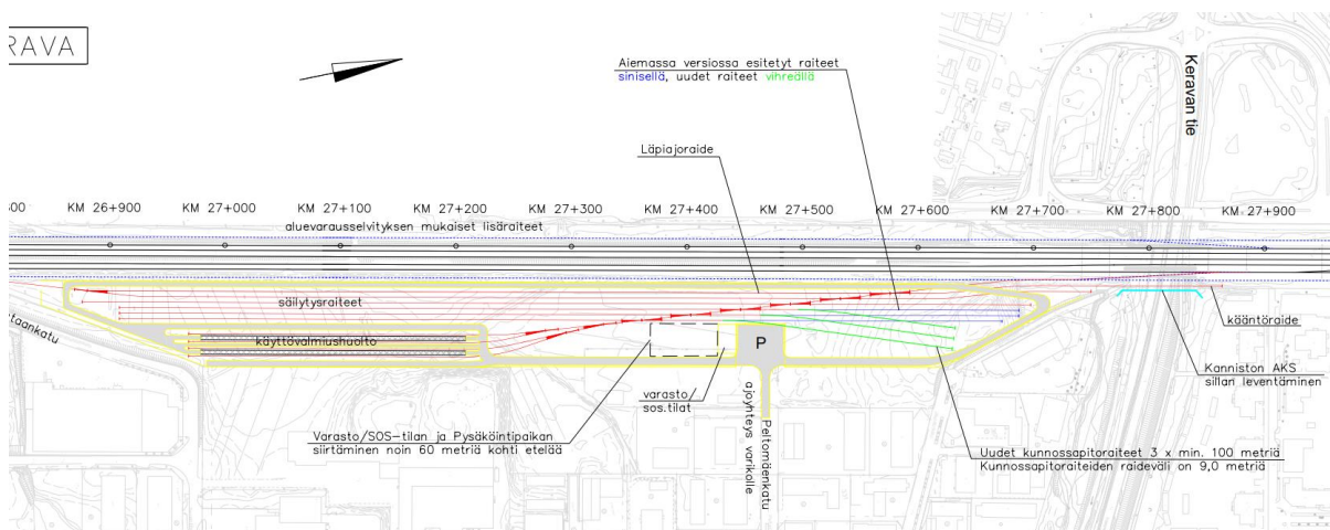
Kuva 13. Alustava suunnitelma Jäspilän varikosta.
