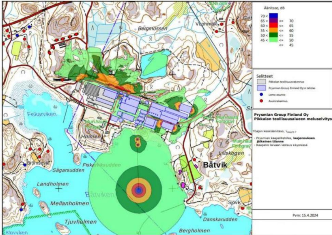
Kuva 6. Kaapelitehtaan toiminnan aiheuttama melu laajennuksen jälkeen, kun kaapelin alukseen lastaus on käynnissä, yöajan keskiäänitasona L_{eq} 22-7 .
