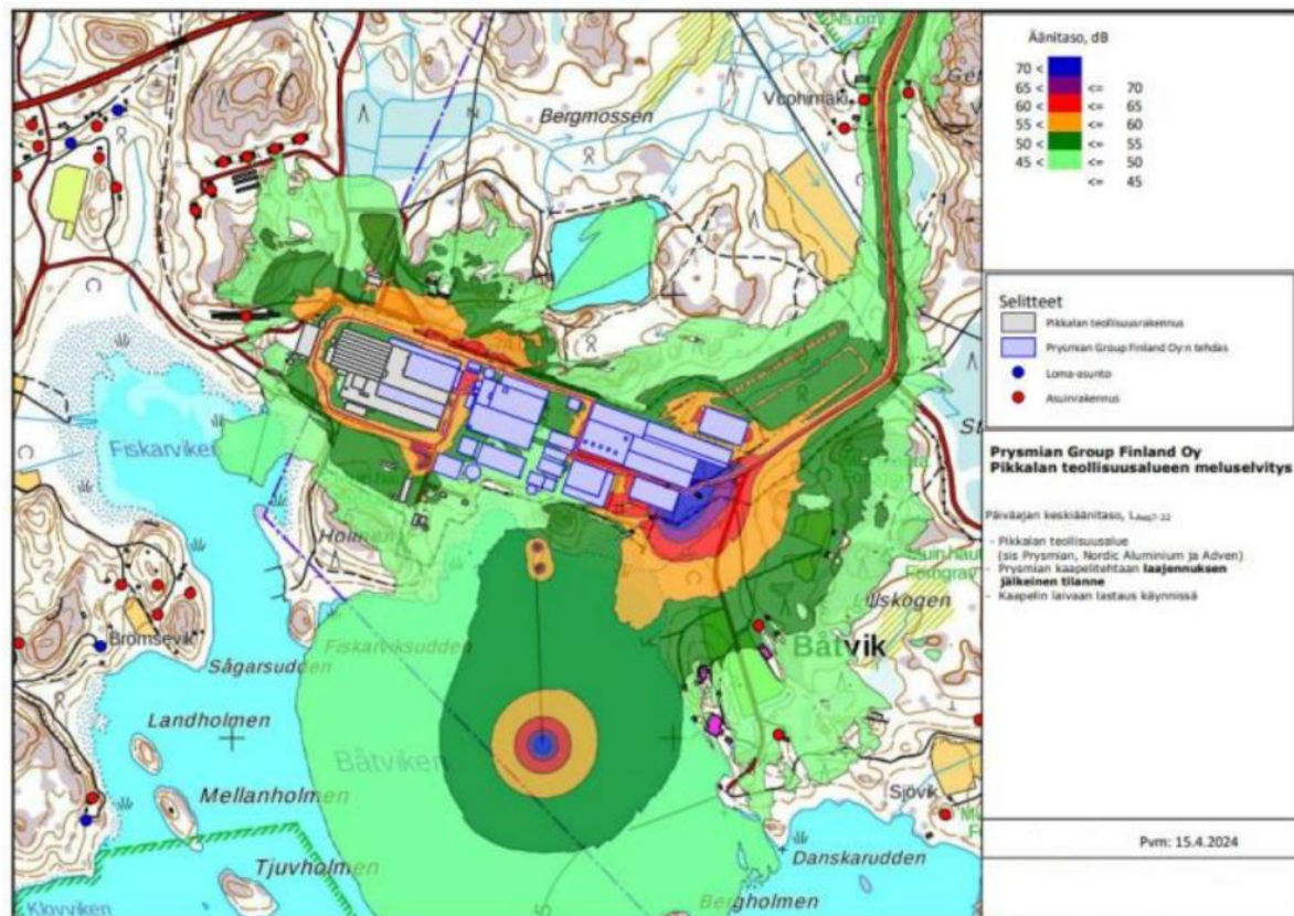
Kuva 5. Kaapelitehtaan toiminnan aiheuttama melu laajennuksen jälkeen, kun kaapelin alukseen lastaus on käynnissä, päiväajan keskiäänitaso L_{eq,T=22} .
